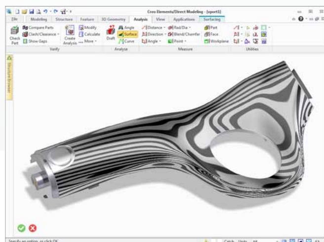
Dynamische Flächenanalyse und Krümmungsvisualisierung mit Creo Elements/Direct Surfacing
